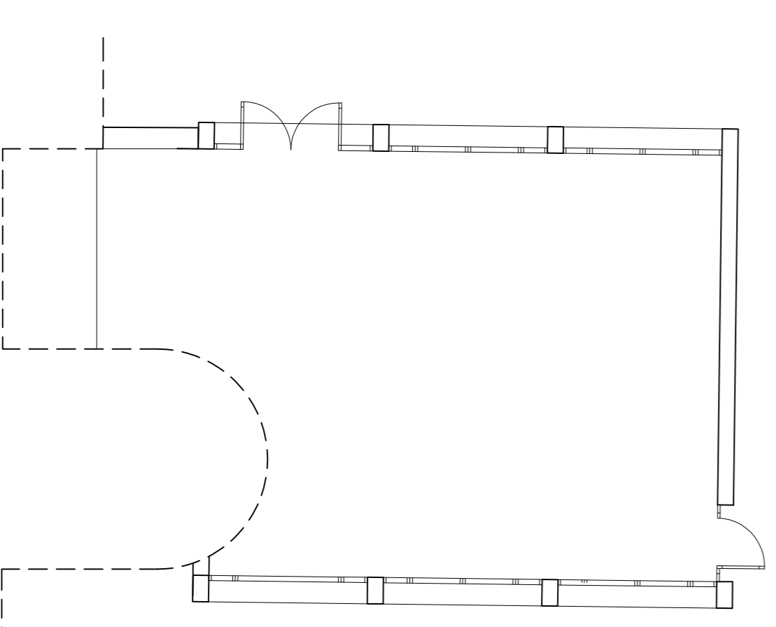
PLANIMETRIA PORTICATO ESTERNO COPERTO (C) PIANO TERRA 1:100
